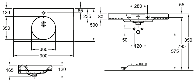
PRECIOSA II WASCHTISCH CE, EN 14688 CL 25 900 x 500 mm Modell-Nr. 123290
