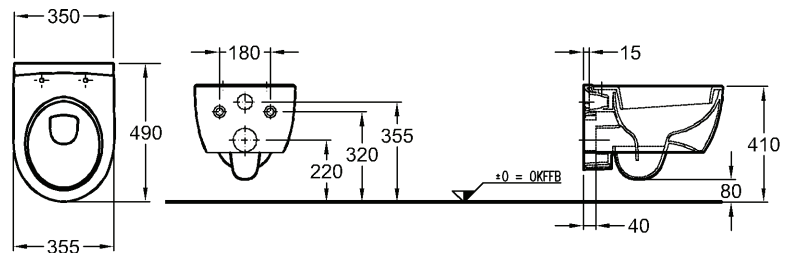
4U TIEFSPÜL-WC wandhängend kurze Ausladung (490 mm) CE, EN 997 6 A/C, EN 38 Modell-Nr. 203430
