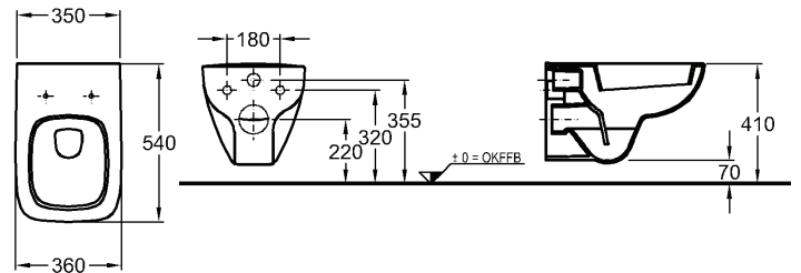
RENOVA NR. 1 PLANTIEFSPÜL-WC wandhängend CE, EN 997 6 AC/5 A, EN 38 Modell-Nr. 202150
